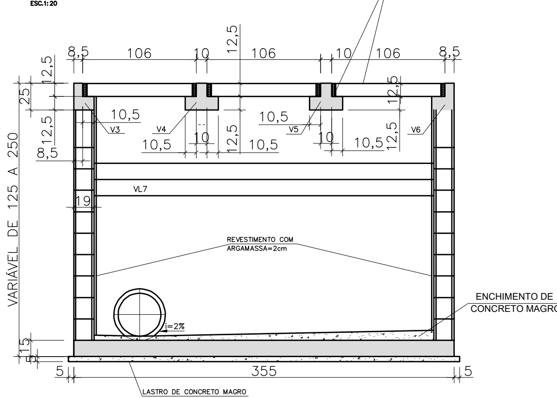
CORTE A-A
