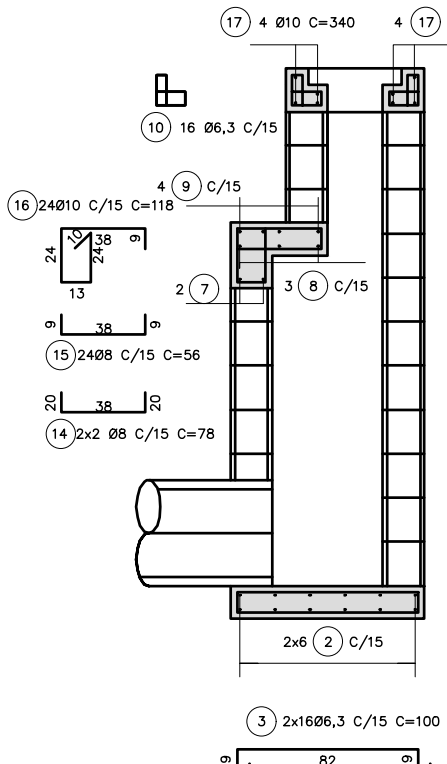
CORTE B-B-ARMAÇÃO
