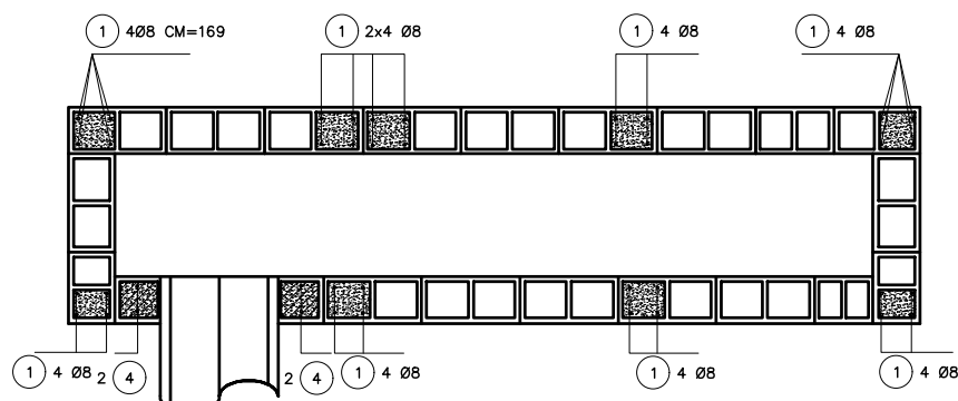
PLANTA – ARMAÇÃO
