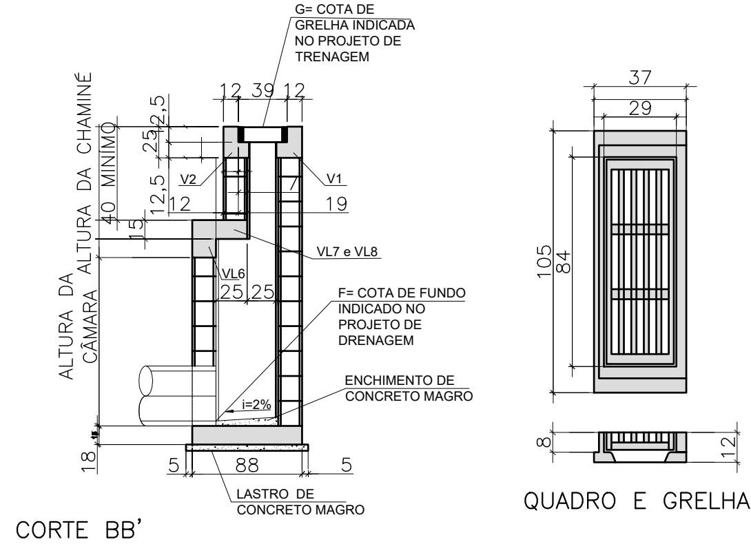
CORTE BB'
