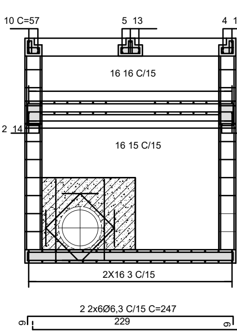
CORTE AA' – ARMAÇÃO
