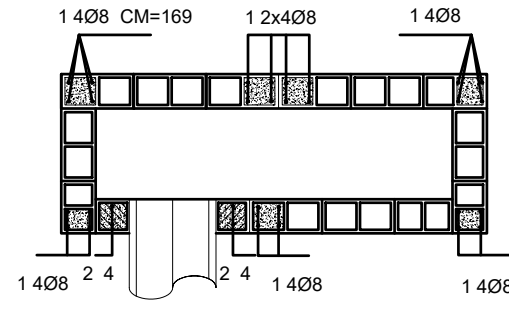
PLANTA – ARMAÇÃO
