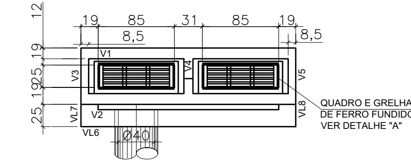
PLANTA SUPERIOR
