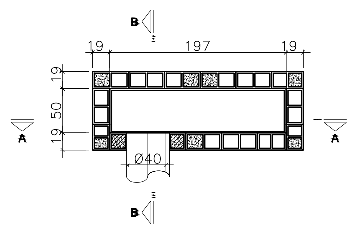
PLANTA INFERIOR
