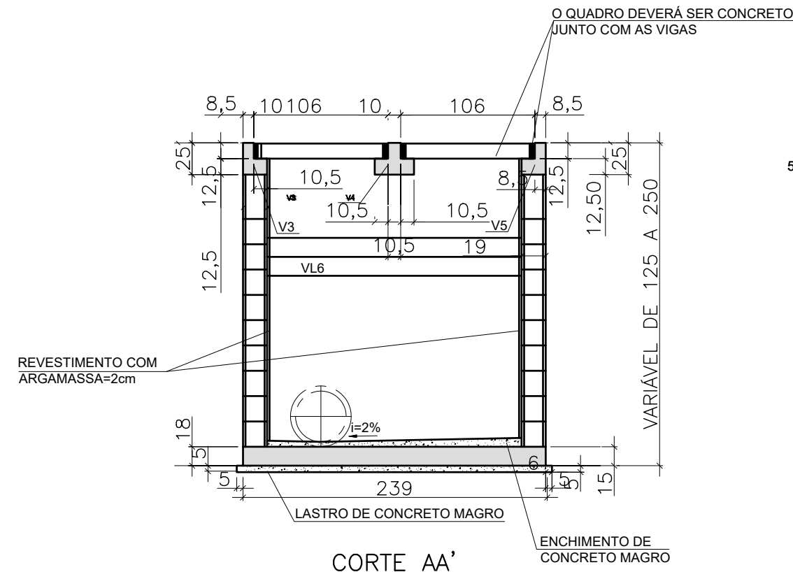
CORTE AA'
