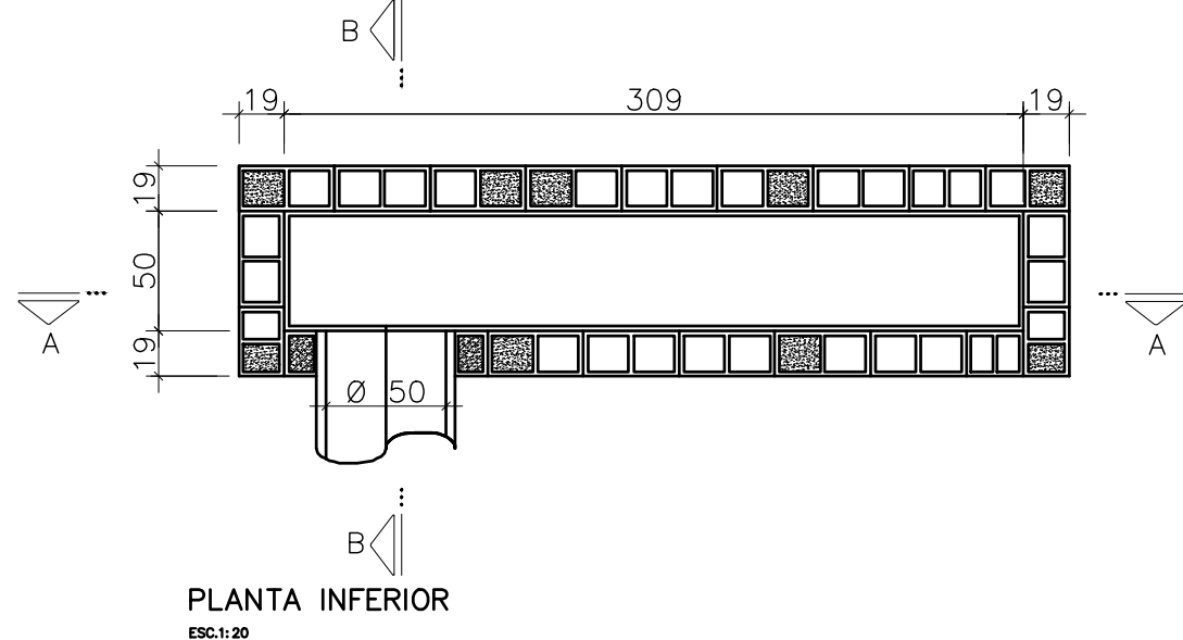
PLANTA INFERIOR
