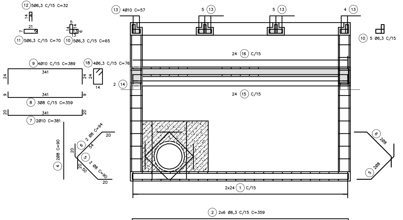
CORTE A-A-ARMAÇÃO
