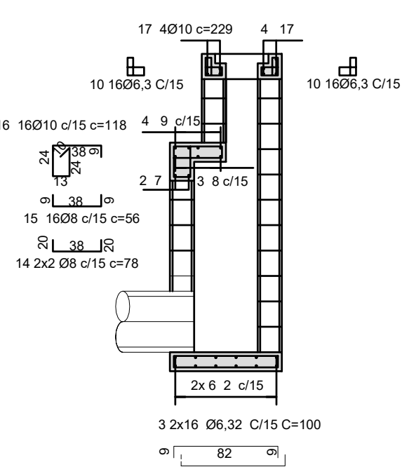
CORTE BB' – ARMAÇÃO
