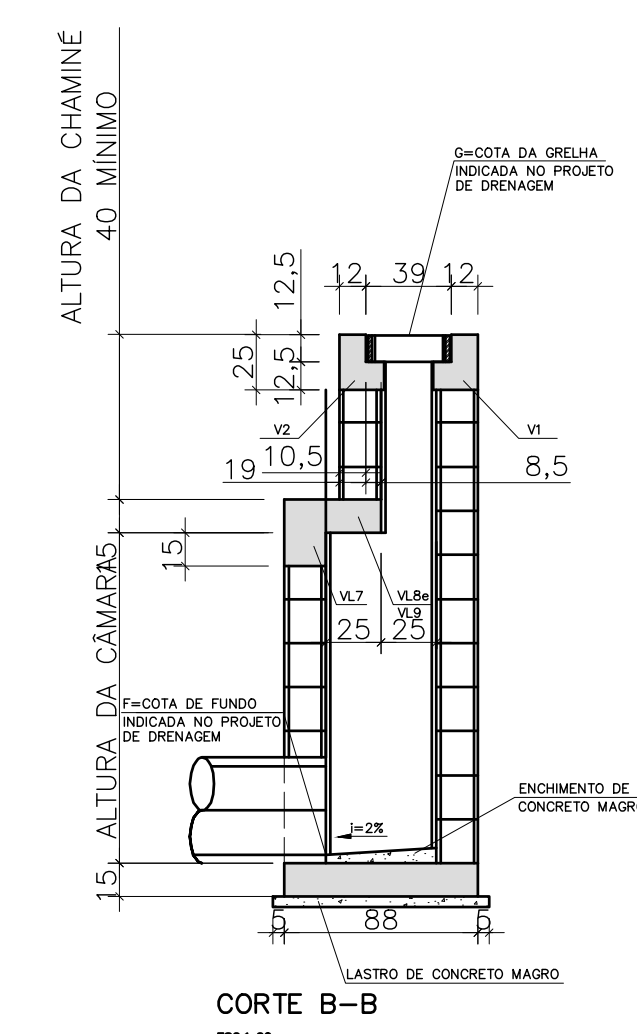
CORTE B-B
