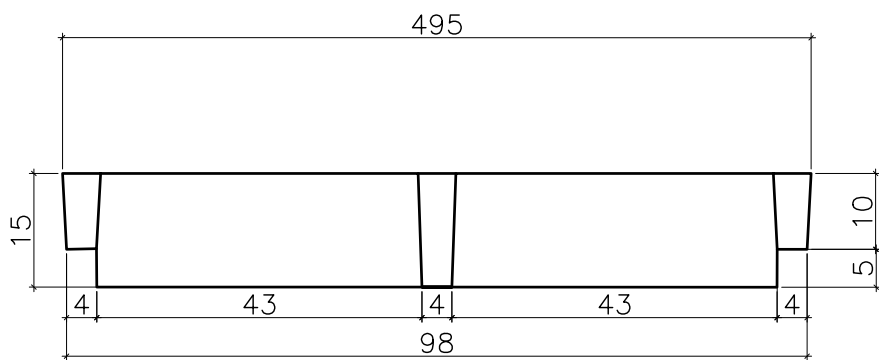
CORTE AA – TIPO B
