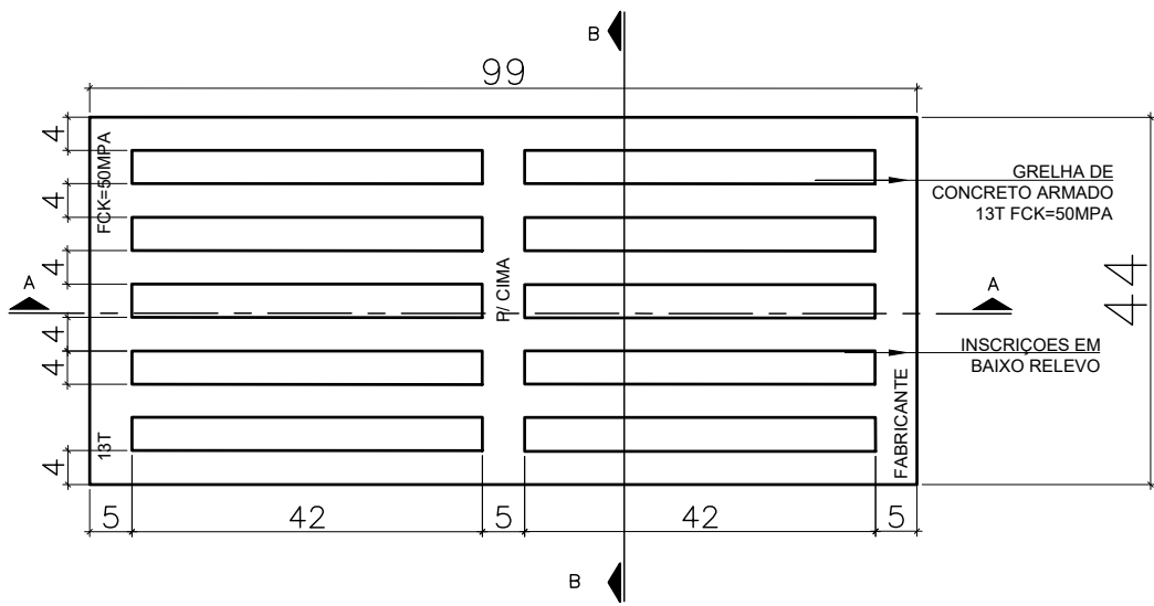
PLANTA BAIXA – GELHA B
