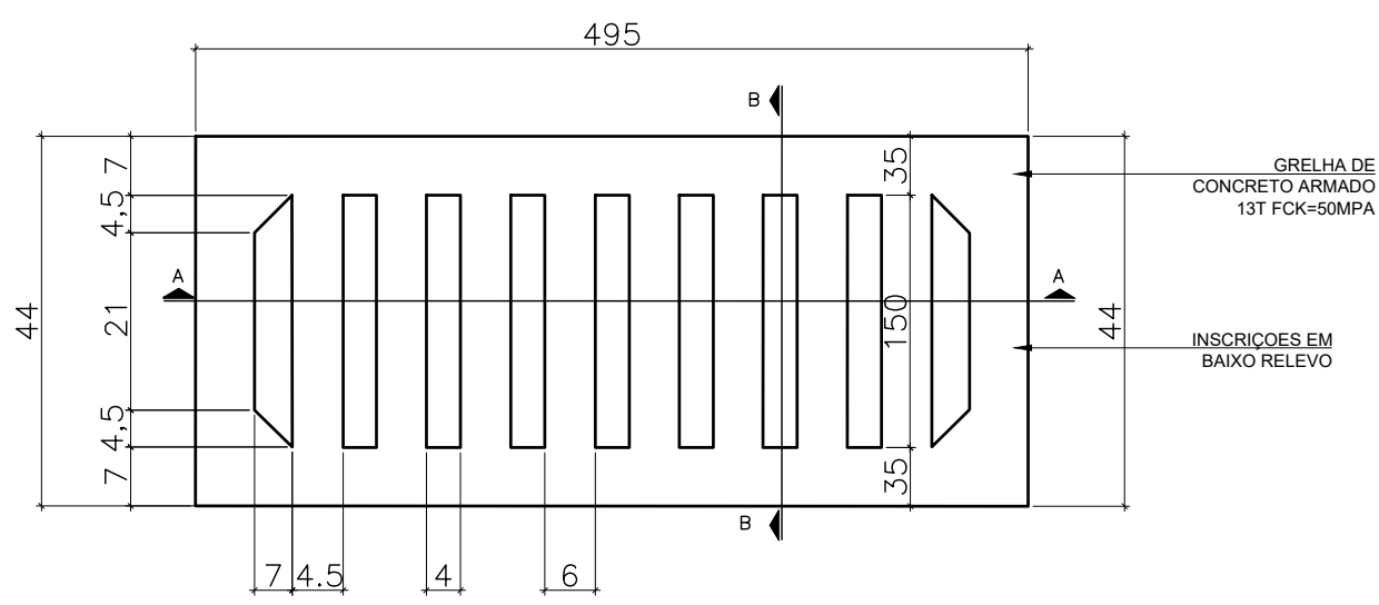
PLANTA BAIXA – GELHA C
