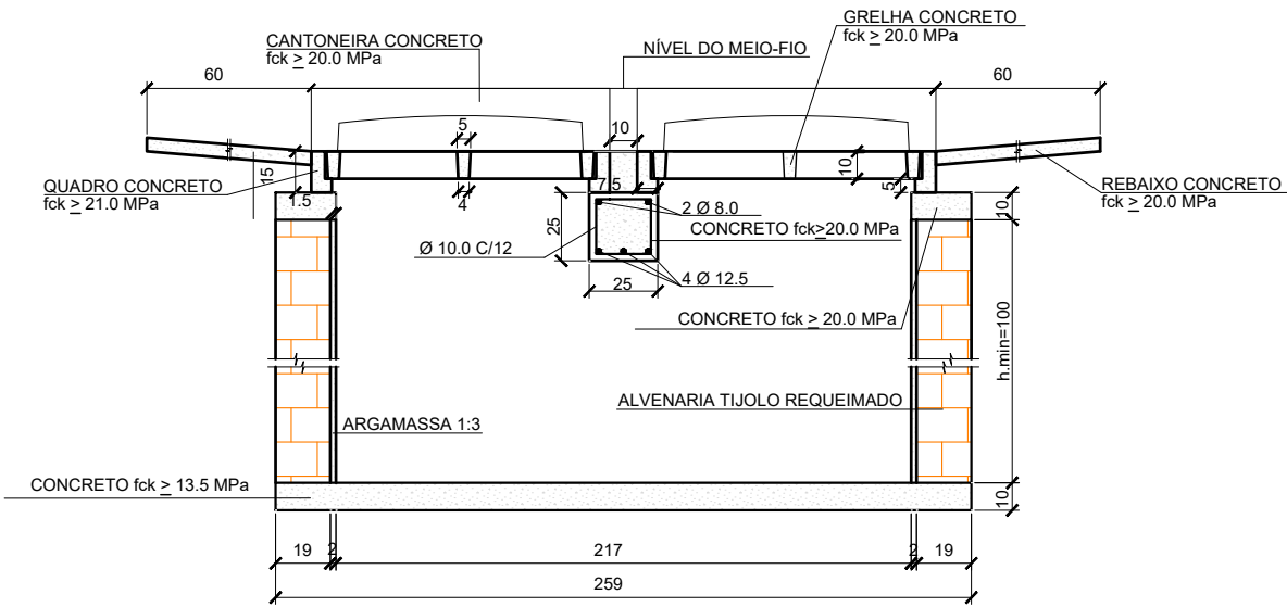
VISTA LATERAL
